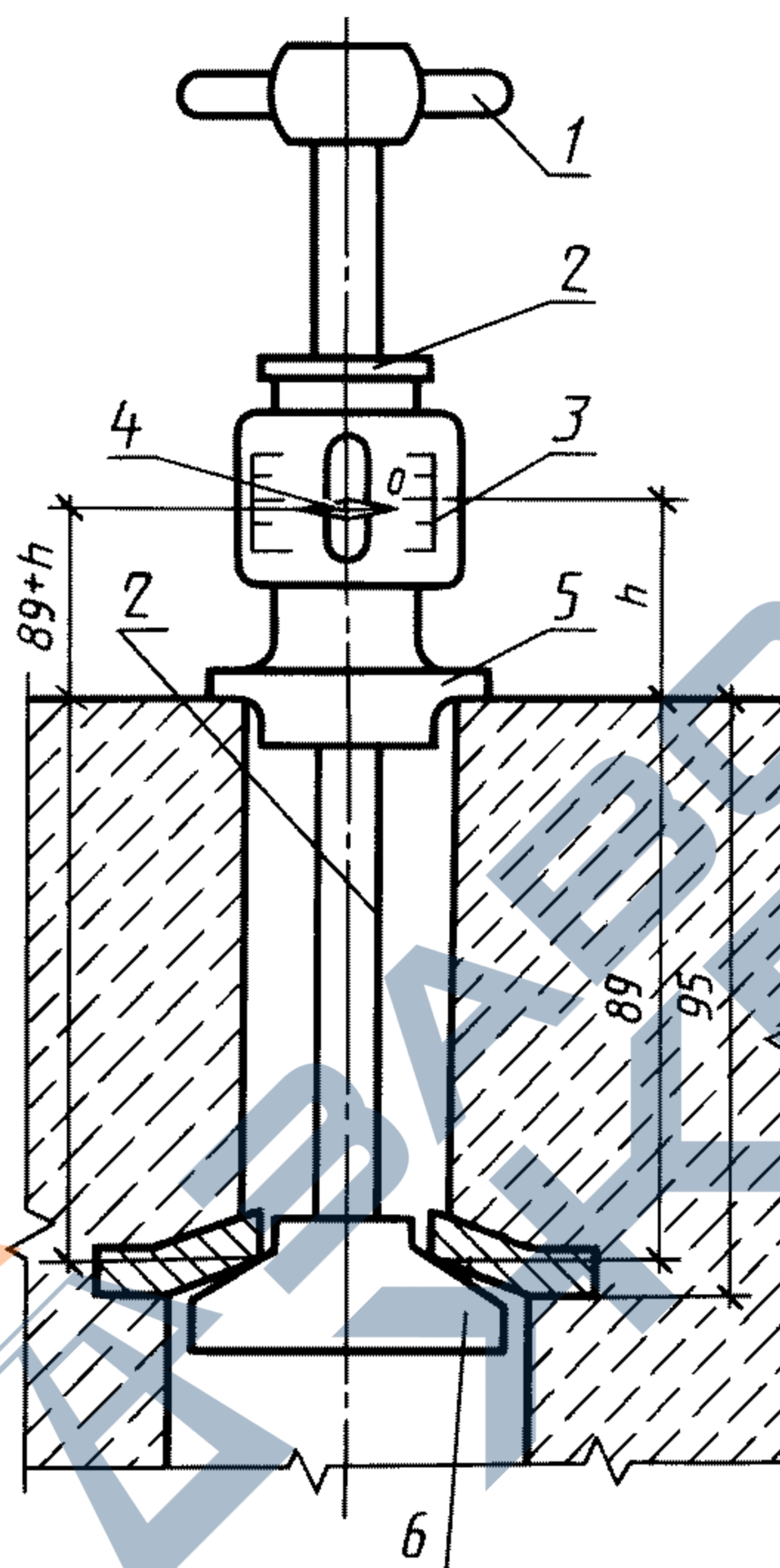
1 — ручка; 2 — шток; 3 — шкала; 4 — указатель; 5 — корпус; 6 — головка
