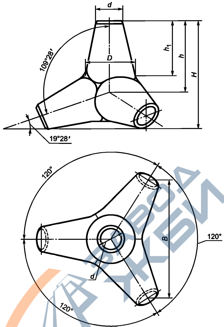
Рисунок 1 — Тетрапод
